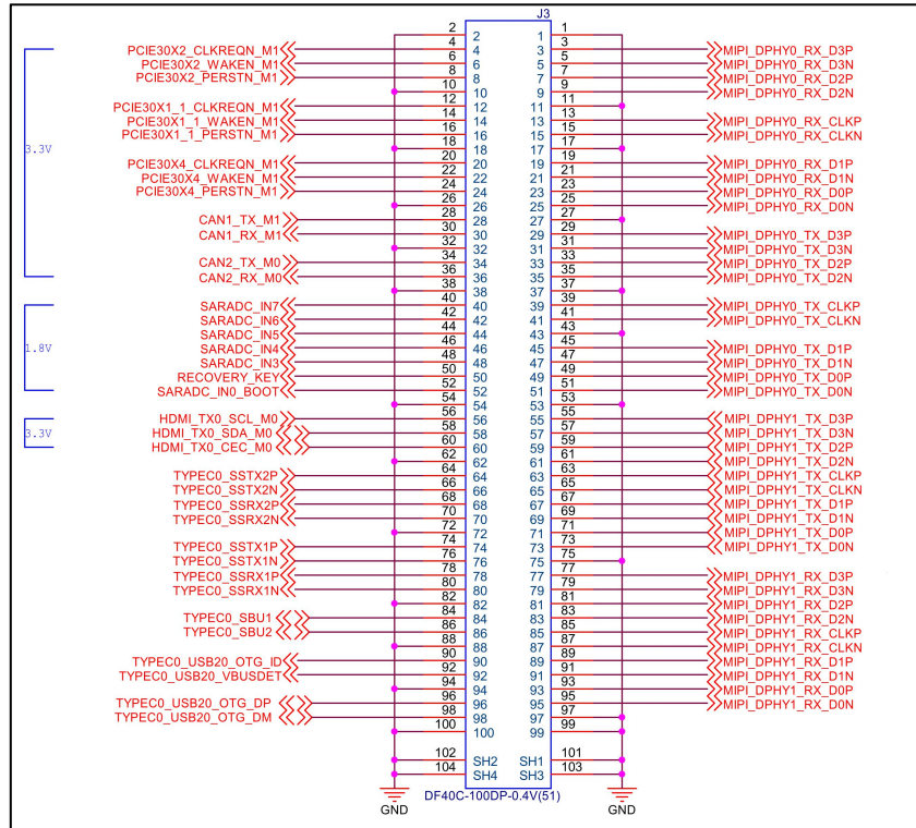
图 4.6-3 J3 连接原理图
